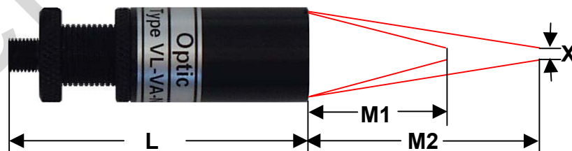
可调焦镜头 Ø 18mm
